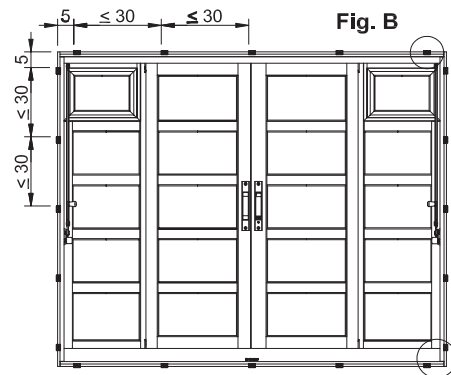
Det.3 Vista interna do ambiente
