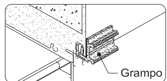
Det.2 Vista lateral em corte
