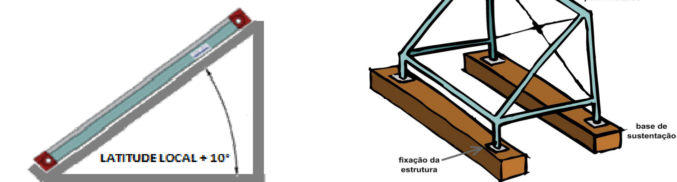
Figura 14 – Suporte de Sustentação das Placas Coletoras
