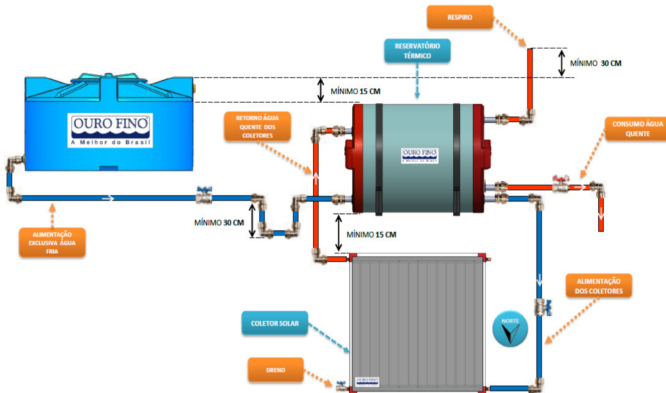
Figura 26 – Exemplo: Esquema Reservatório baixa pressão em nível - Sistema Termossifão
