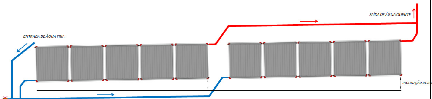
Figura 16 – Baterias em paralelo
